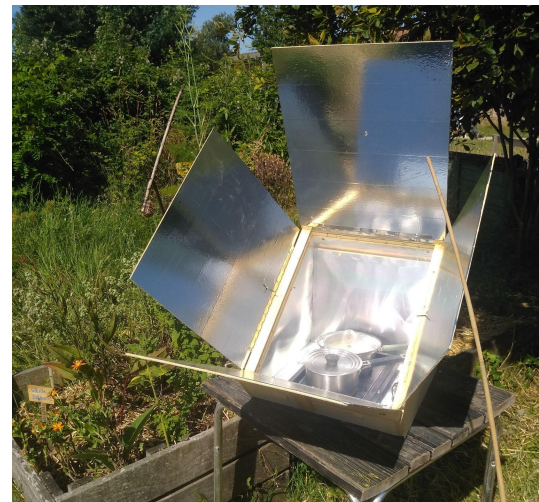
Four solaire
